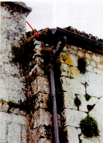
Descente d'eaux pluviales à l'angle entre le clocher et la nef : maçonnerie désorganisée avec pierre manquante, joints dégarnis et végétation abondante liées aux infiltrations en tête de maçonnerie, protection à revoir
